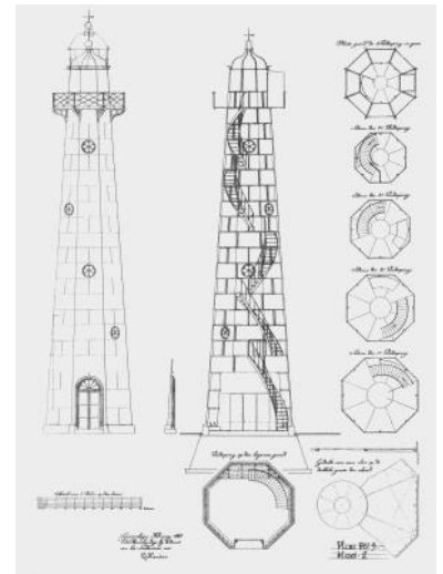
Bestektekning van de vuurtoren uit 1867, van Quirinus Harder.
