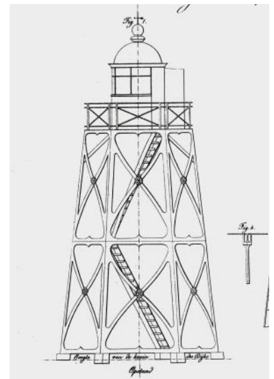
Deel van de bestektekning van het lage licht uit 1867, van Quirinus Harder.
