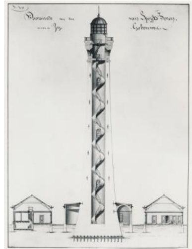
Ontwerp voor de Van-Speijktoeren uit 1833. De toren bestaat uit slechts één cilinder.
