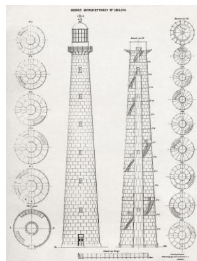
Bestektekening van de vuurtoren van Ameland uit 1880, van Quirinus Harder.
