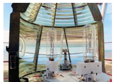
Optiek en lampenwisselaar.
